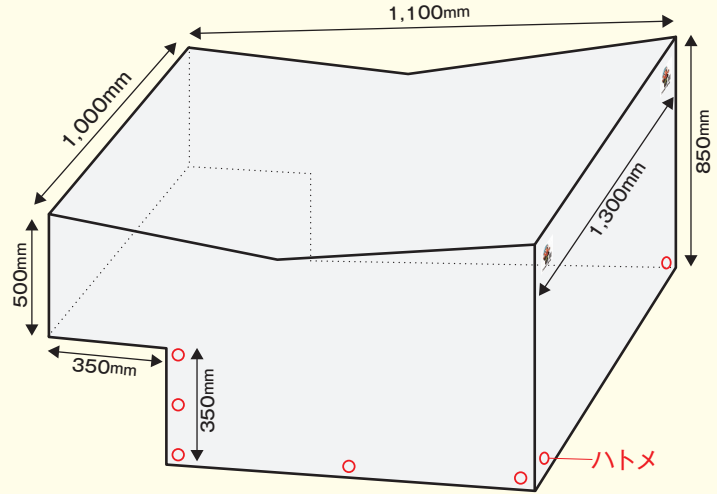
【オールハッピー寸法】
